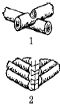
Рубка углов избы: 1 – «в обло»; 2 – «в лапу»
