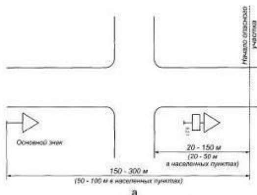
Рис.2. Установка предупреждающих дорожных знаков: а – между основным знаком и началом опасного участка имеется перекресток
