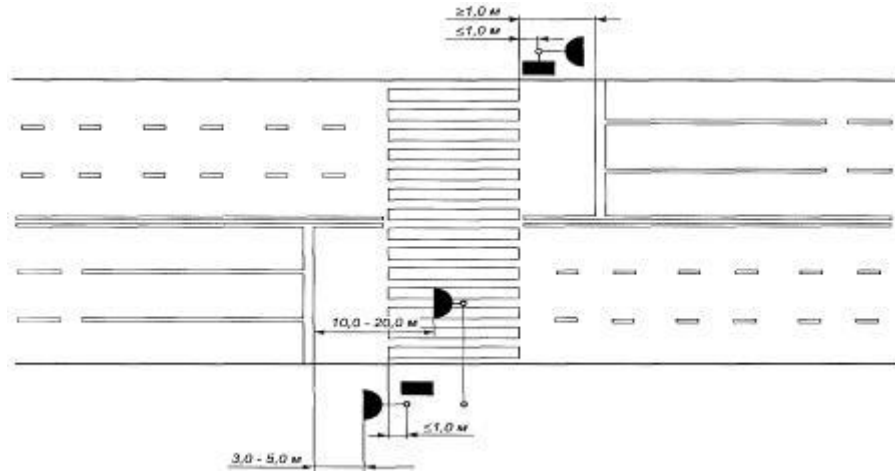
Рис. 5 Пример размещения светофоров и нанесения разметки на регулируемом пешеходном переходе.
